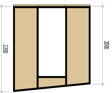
Element 3: Giebelwand mit Türe
